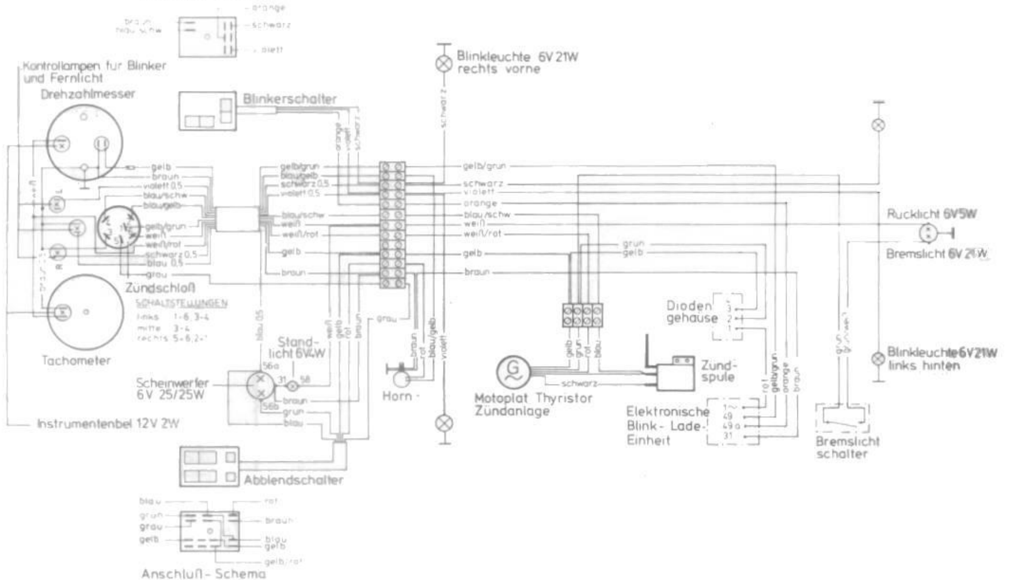
Anschluß - Schema
